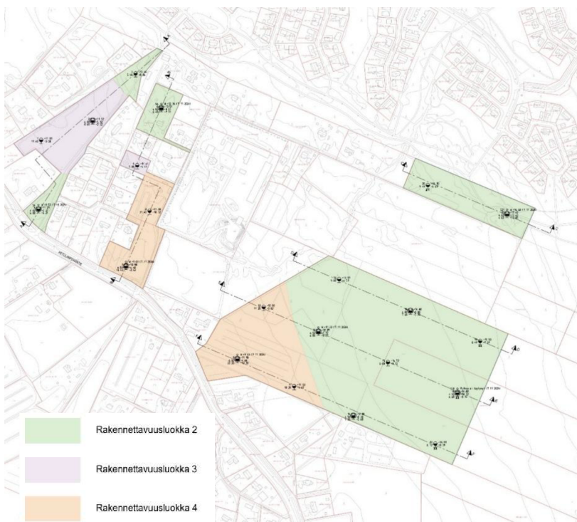
Kuva 8 kaava-alueen rakennettavuusluokat
