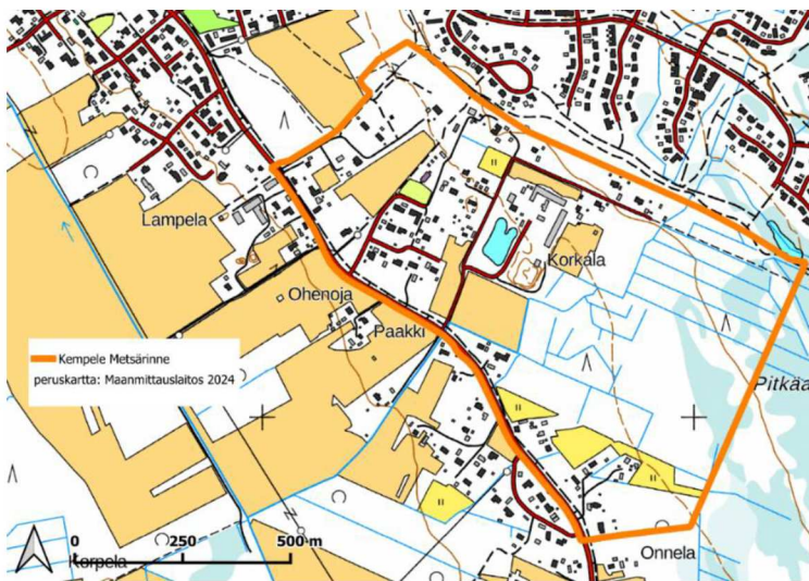
Kuva 5 lepakkoselvityksen selvitysalue
