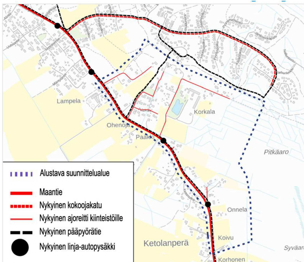
Kuva 10 Liikenneverkon nykytila
